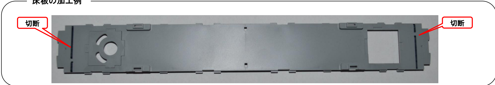
床板の加工例
